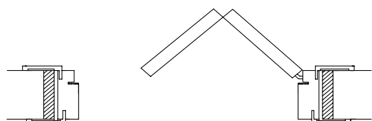
Libro simmetrica Symmetrical fold door pag.36
